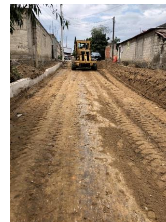
AFINE DE TERRENO NATURAL CON EQUIPO MECANICO
